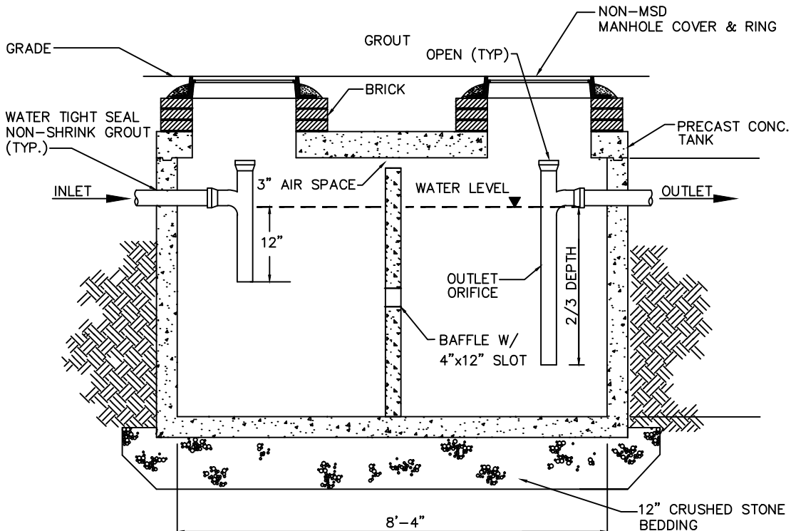
SECTION N.T.S.
