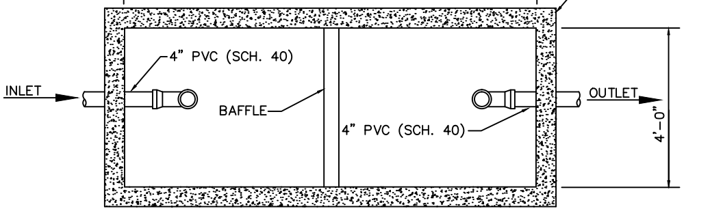
PLAN N.T.S.
